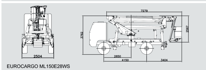
EUROCARGO ML150E28WS
